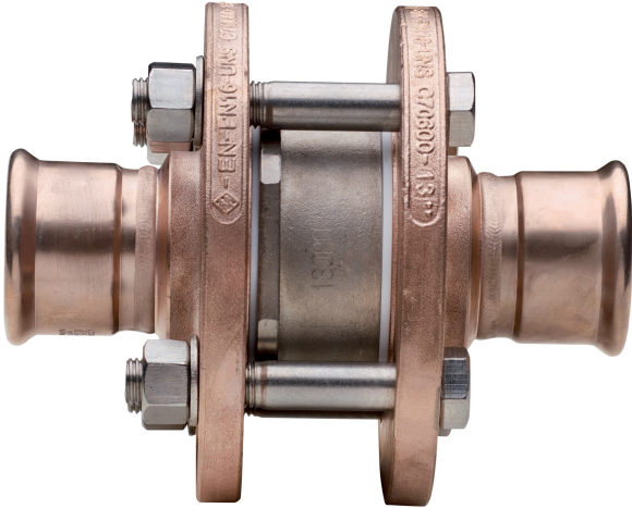
Disco-Rückschlagventil PN16.
